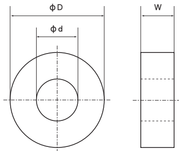
磁芯外径: φ D 磁芯内径: φ d 磁芯宽度: W
